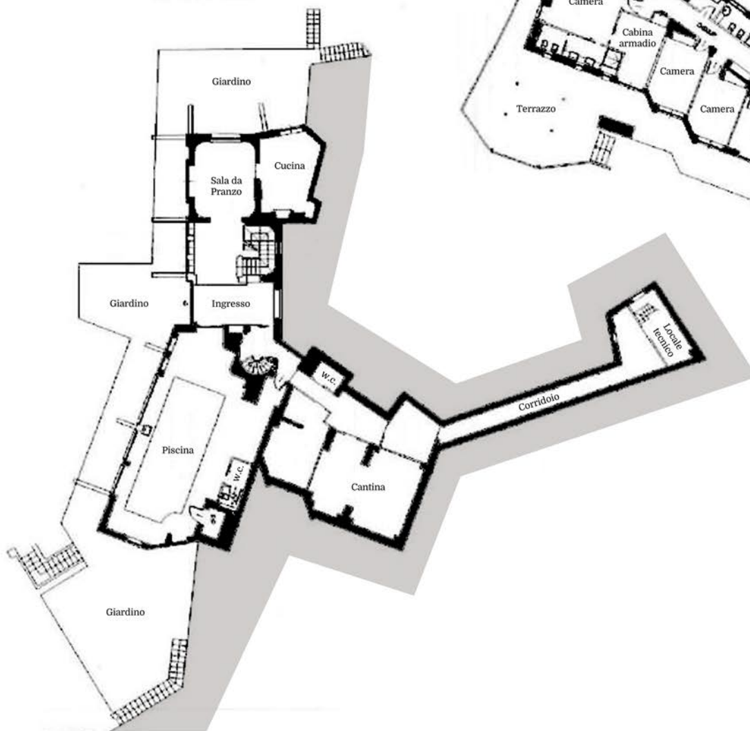
PIANTA PIANO SEMINTERRATO H=300 cm.
